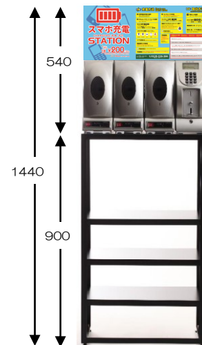
● Gラックサイズ W590 × H900 × D400
